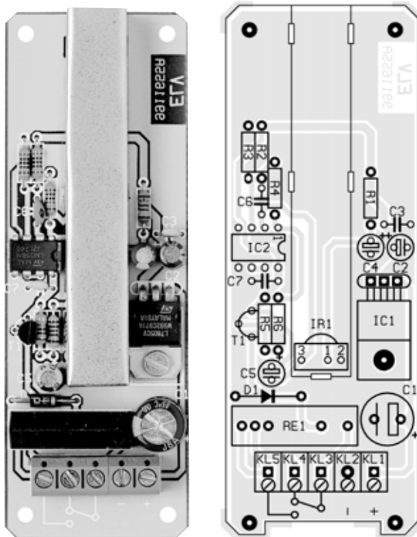
Ansicht der fertig bestückten Empfänger-Platine mit zugehörigem Bestückungsplan
