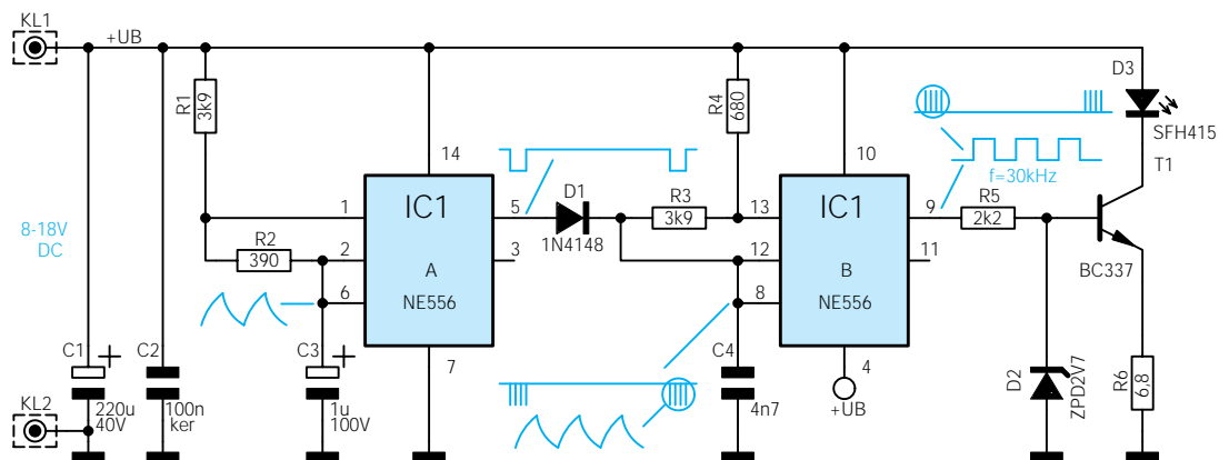
Bild 2: Schaltbild des IR-Senders
