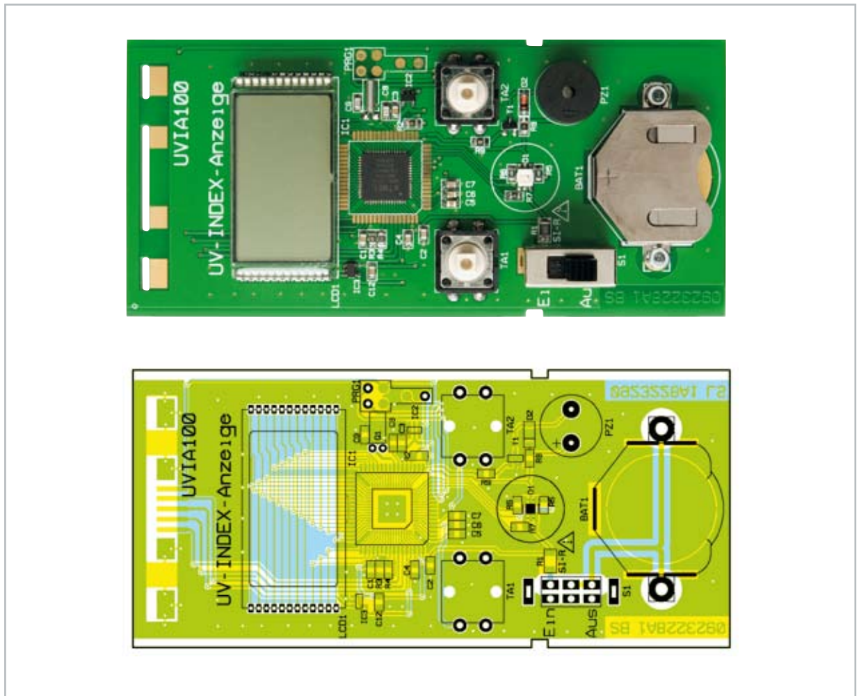
Basiseinheit: fertig bestückte Platine mit Bestückungsplan von der SMD-Seite
