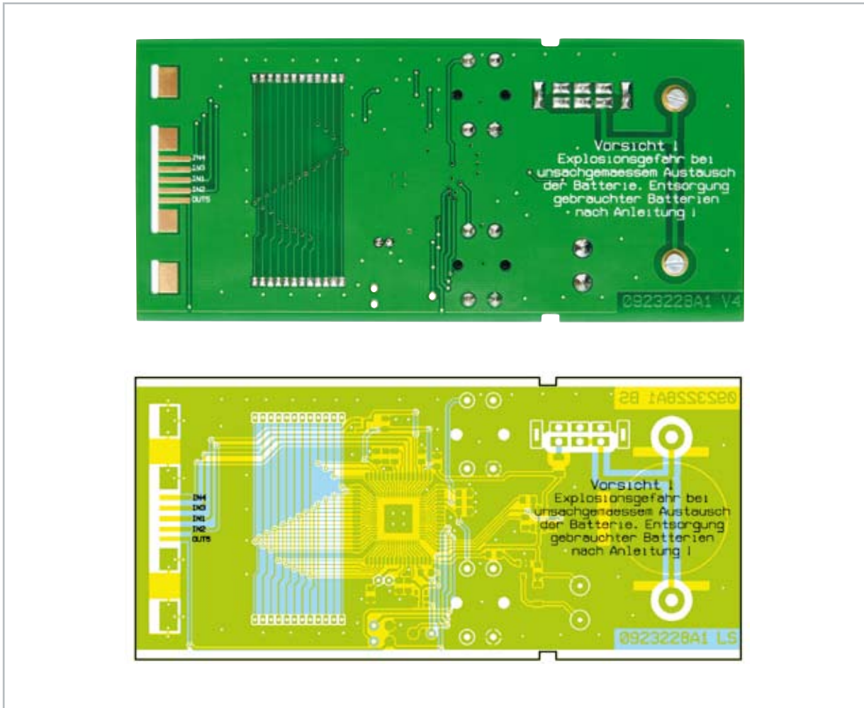
Basiseinheit: die fertig bestückte Platine mit Bestückungsplan von der Unterseite
