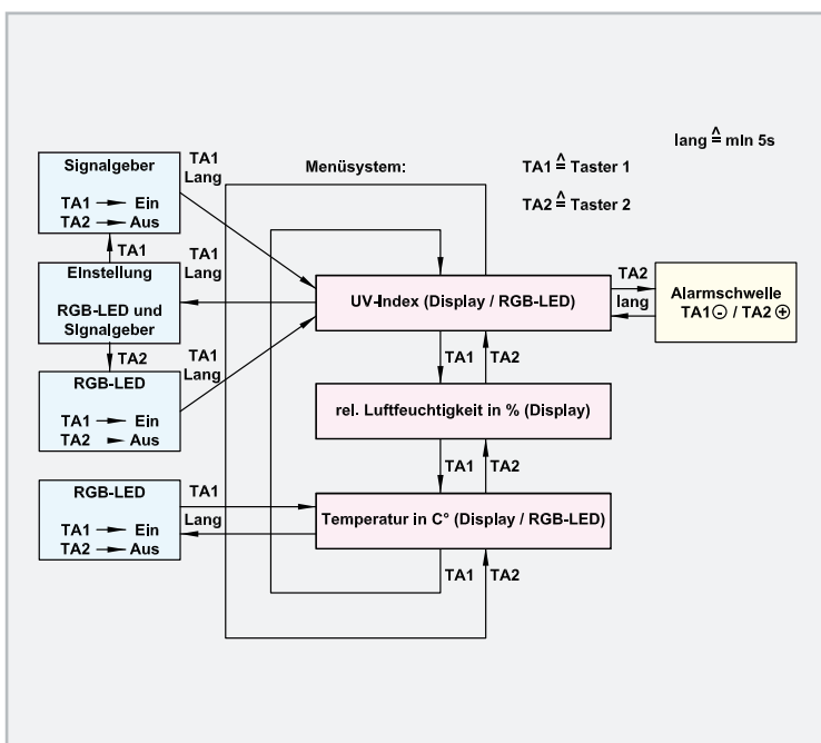
Bild 3: Die Menüübersicht über die Bedienung des UVIA 100
