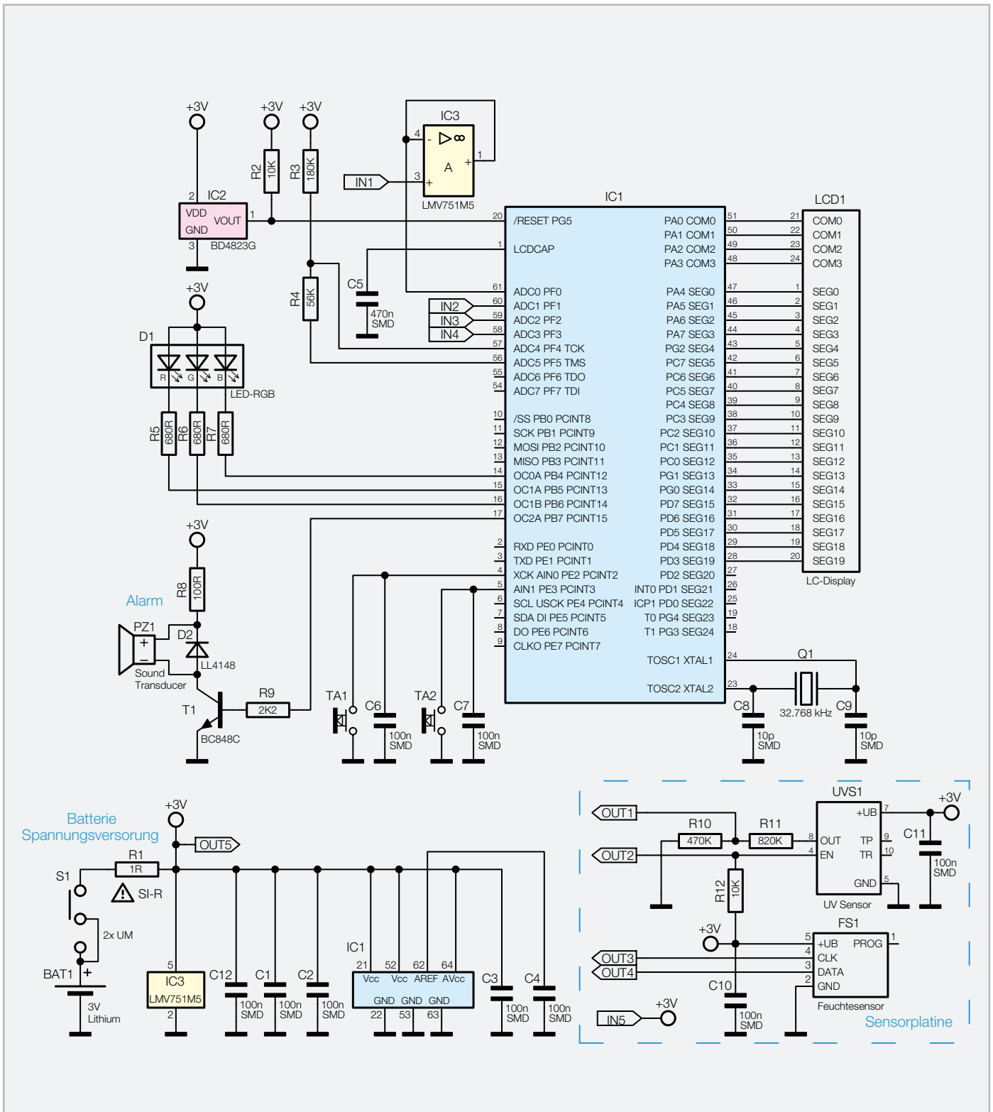
Bild 4: Das Schaltbild des UV-Index-Anzeigegerätes
