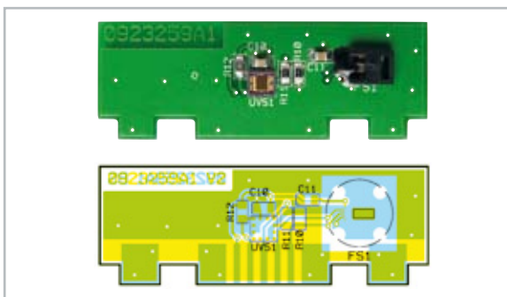
Fertig bestückte Sensoreinheit
