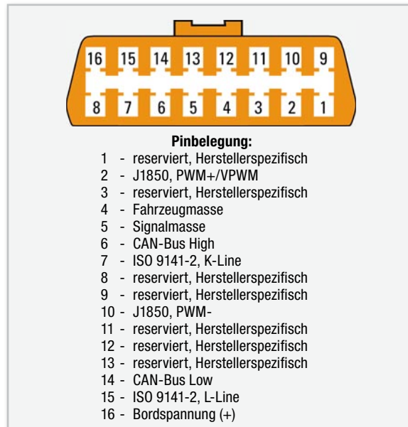
Bild 2: Die Belegung der OBD-II-Buchse im Fahrzeug. Die reservierten Pins können vom jeweiligen Hersteller individuell belegt werden.
